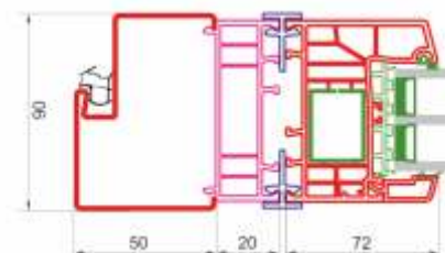
Połączenie NAŚWIETLA PCV z ościeżnicą stalową w linii EKO-NORM oraz PREMIUM (ciepły próg)
