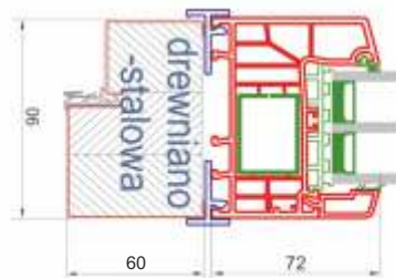
Połączenie NAŚWIETLA PCV z ościeżnicą drewniano-stalową w linii PREMIUM plus oraz TERMO 85
